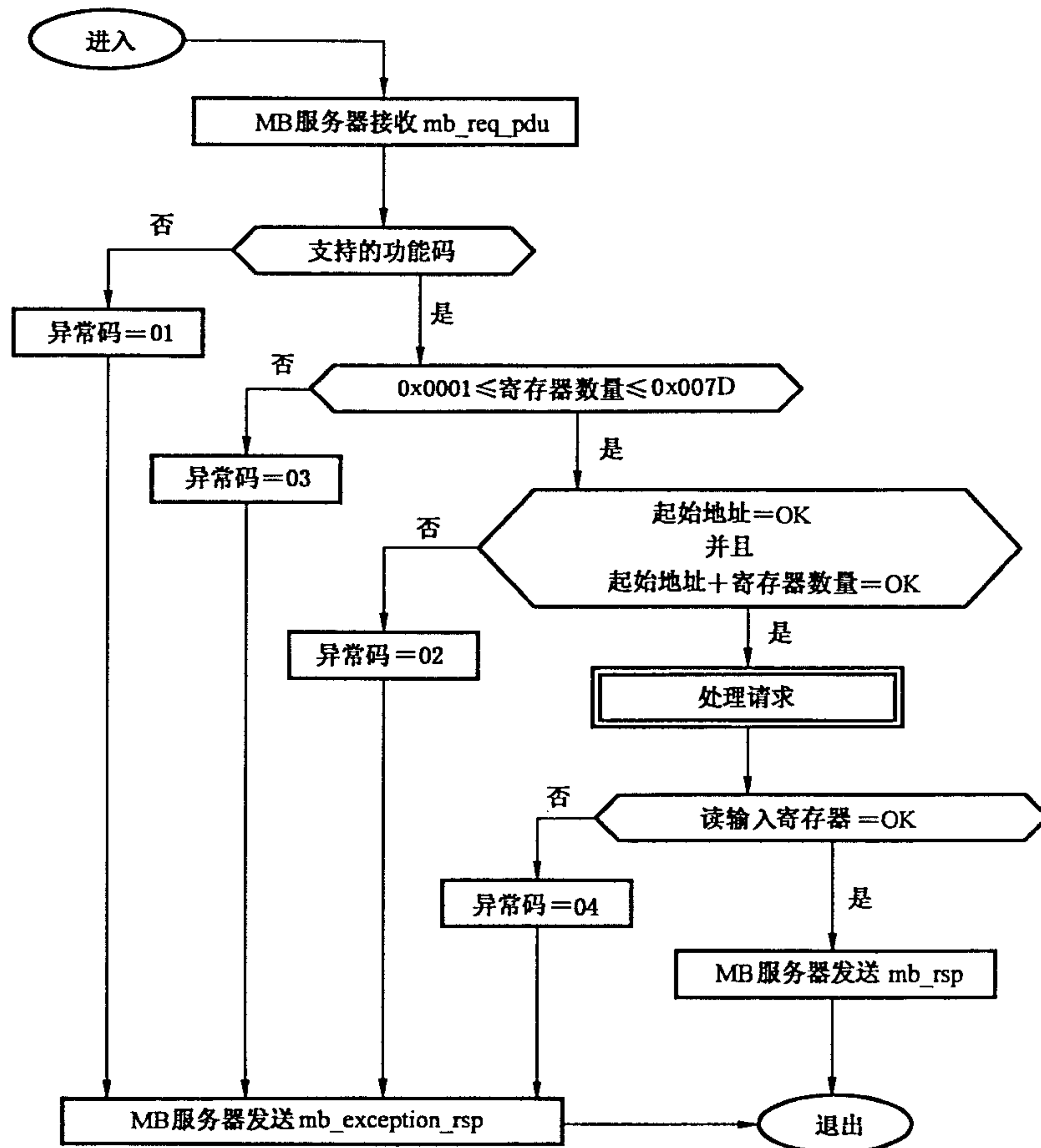
图 14 读输入寄存器的状态图
